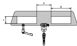
Einfahrtaschen-Innenmaße (Skizze Typ LH-II)
